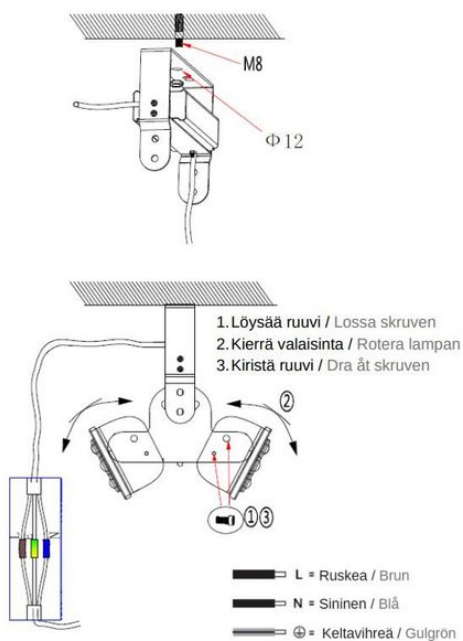
Asennus kattoon / Takinstallation
