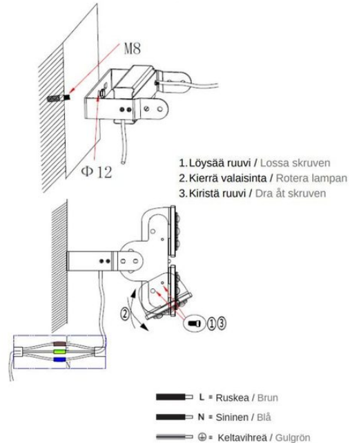
Asennus seinään / Vägghmontering
